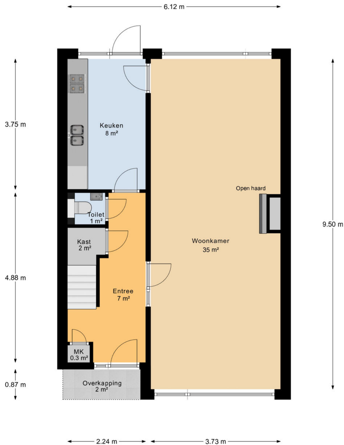
Begane Grond
