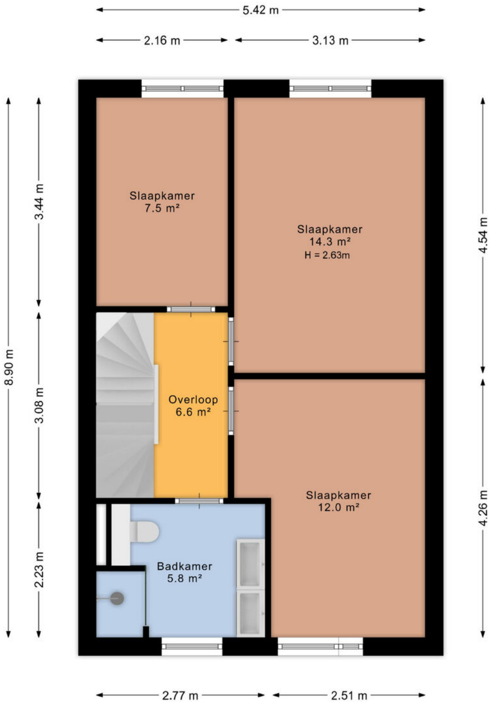
Cella Gallia 44 - Houten Eerste verdieping
