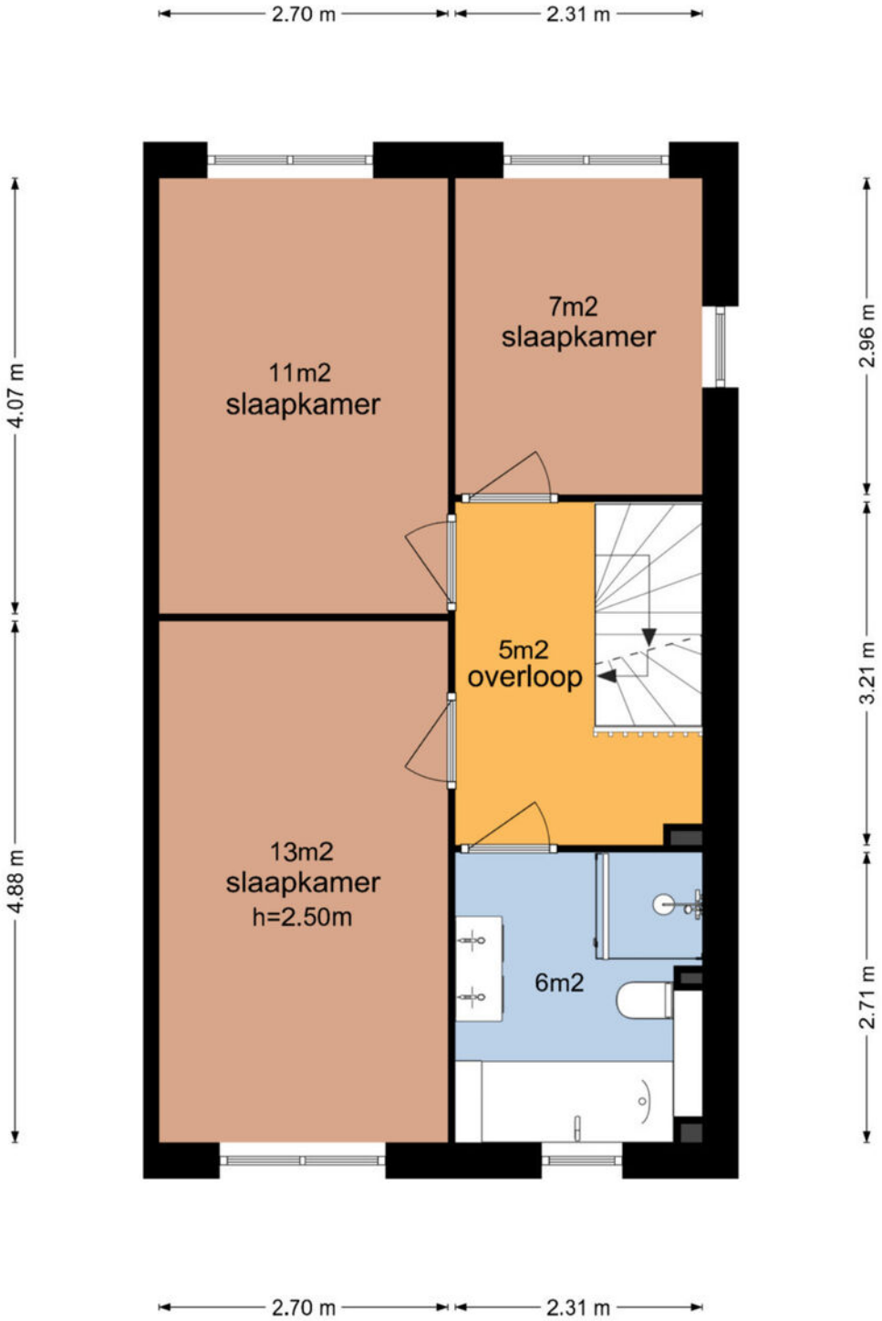
Antonio Morohof 13 - Vleuten Eerste Verdieping
