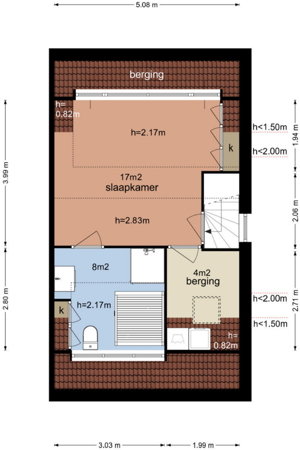
Antonio Morohof 13 - Vleuten Tweede Verdieping
