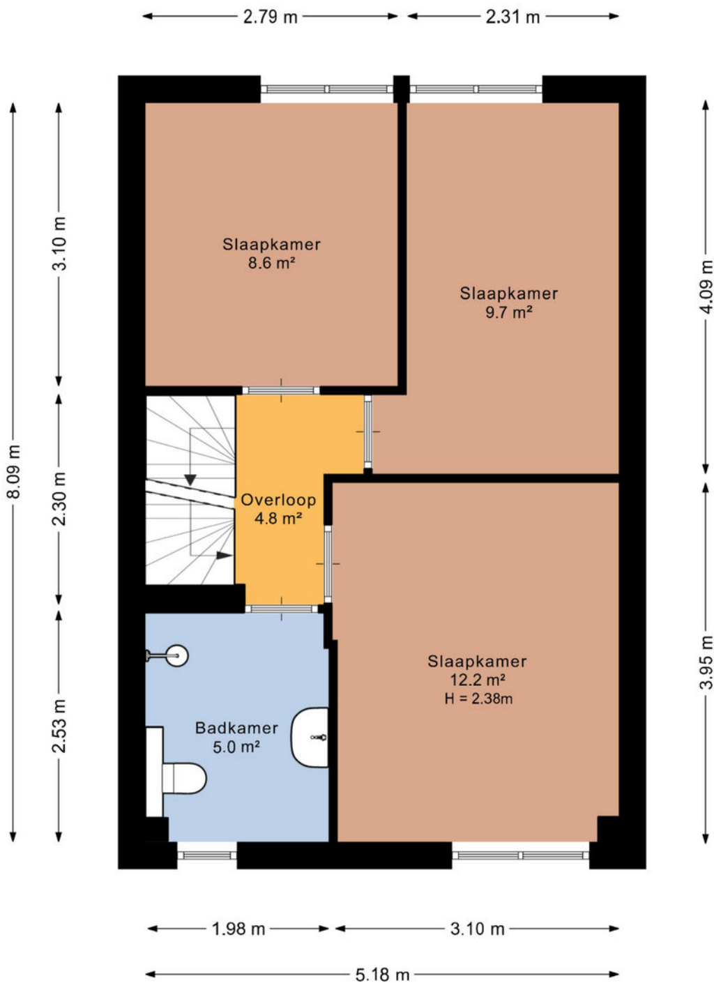
Muiderschans 269 Eerste verdieping
