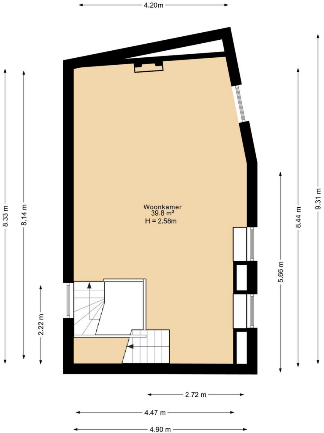
Dorpsstraat 55, Nieuwegein Eerste verdieping
