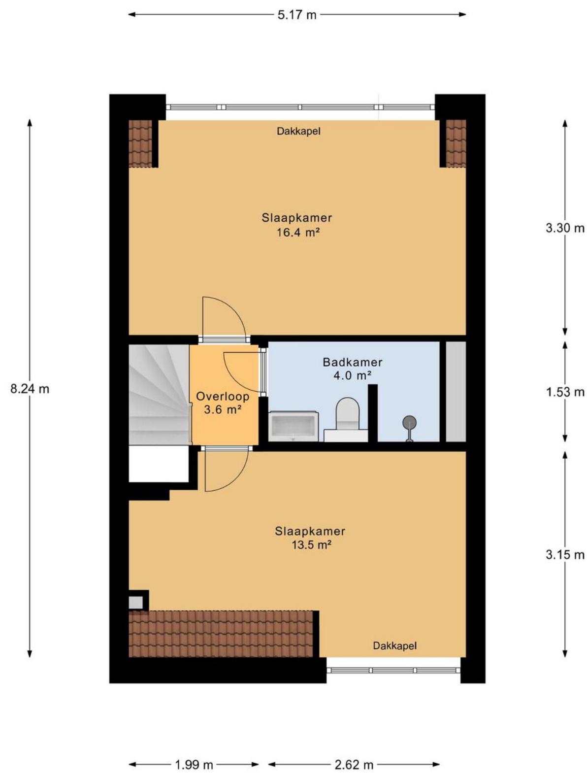
1e Verdieping
