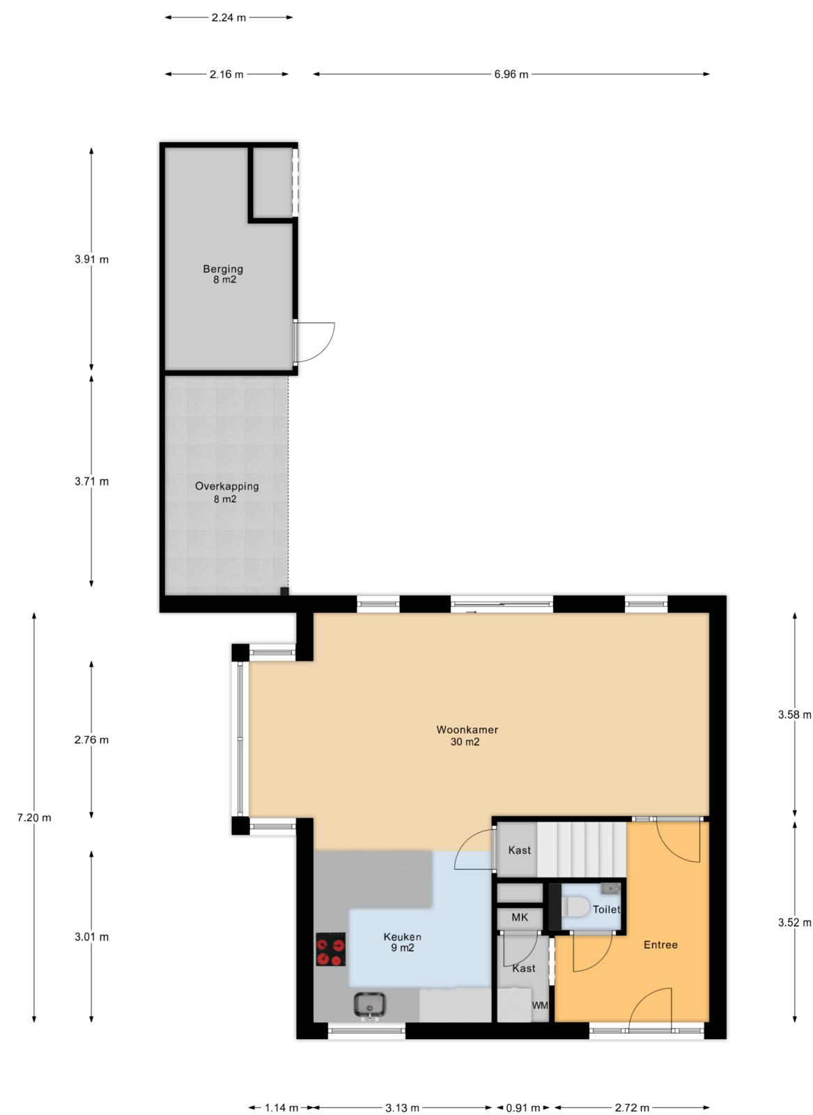
Begane Grond
