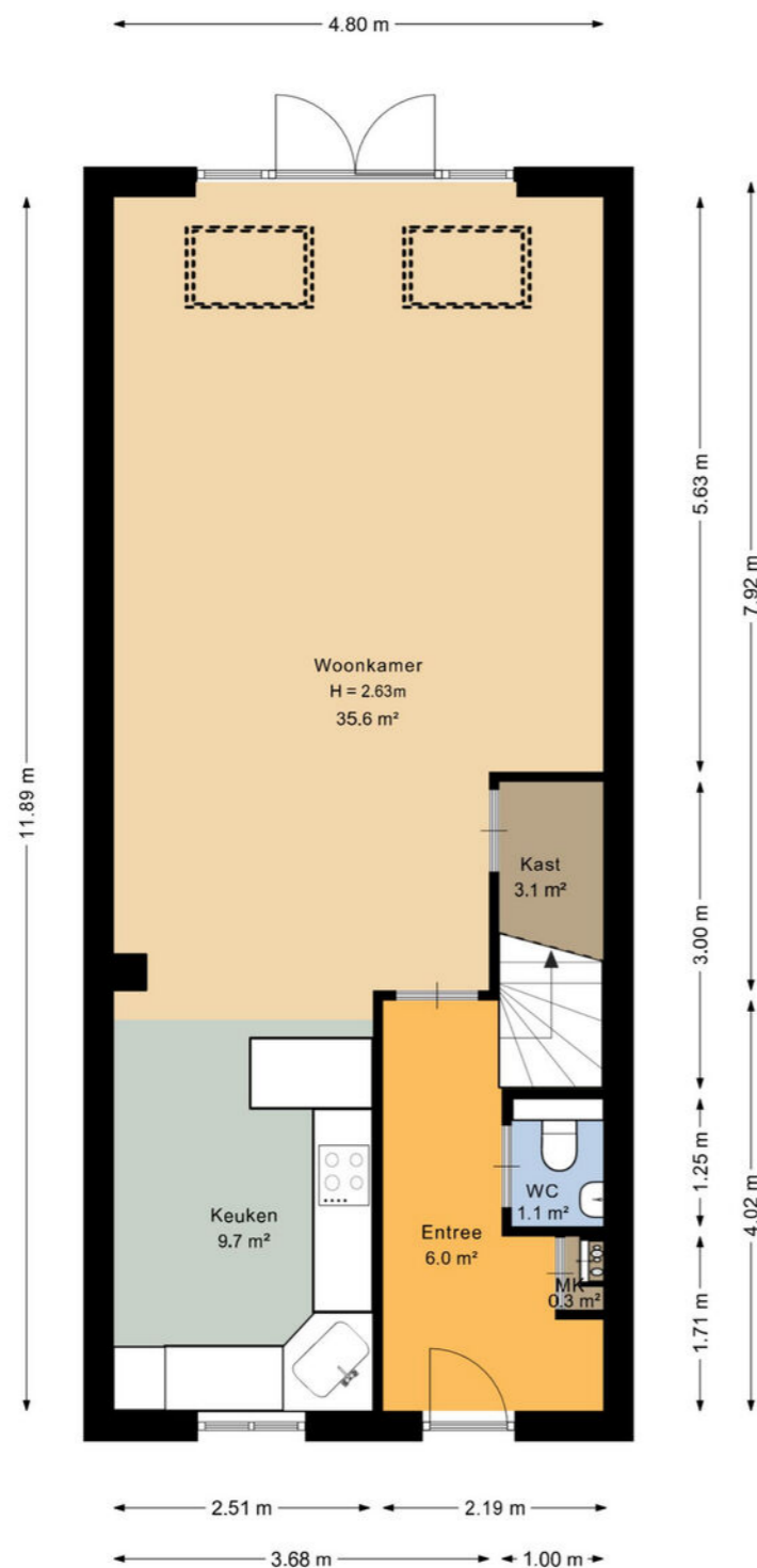
IJzerwerf 6 - Nieuwegein Begane grond
