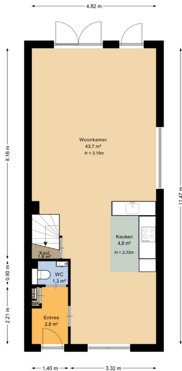
Wijnesteijnstraat 17-1 - Nieuwegein Begane grond
