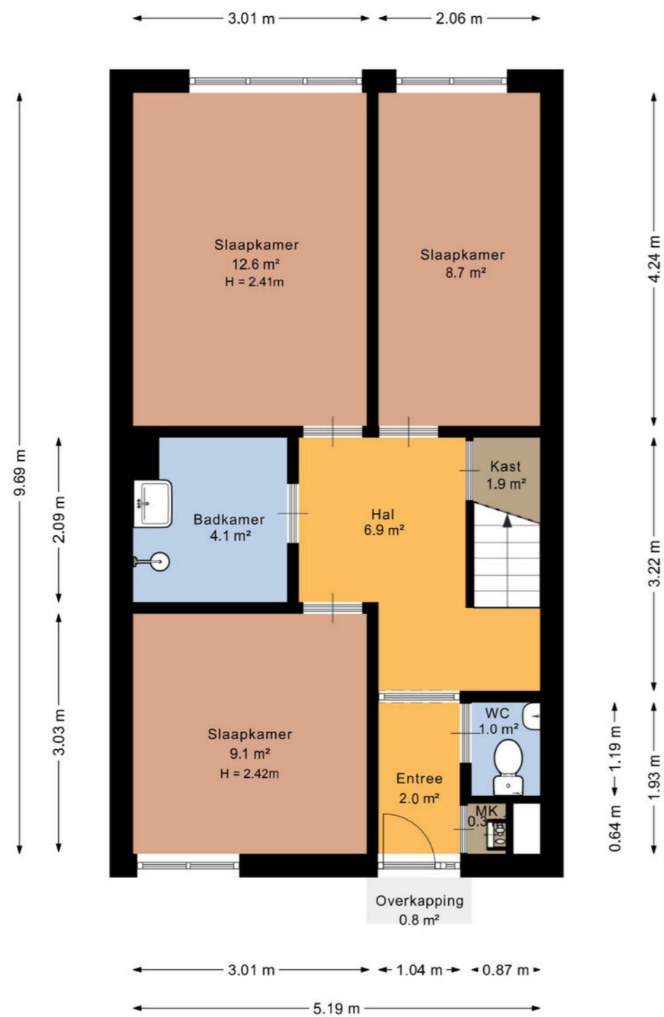
Kloosterdrift 56, Nieuwegein Eerste verdieping
